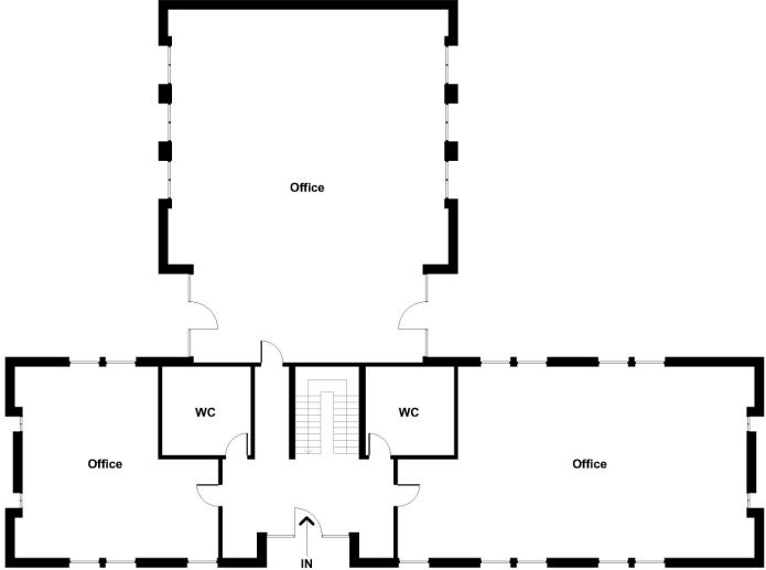
Level 0 - Block 2 Scale: 1:100
